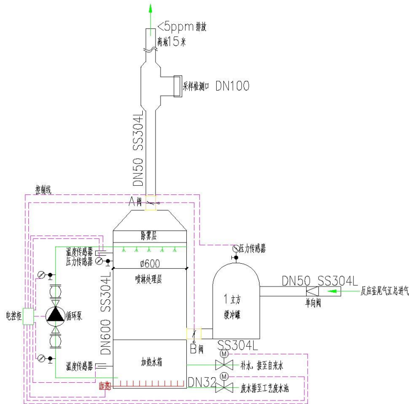
图 4-1 酸液洗涤塔示意图
