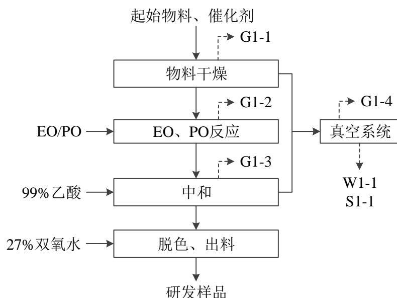
图 2-2 研发实验流程及产污环节图
