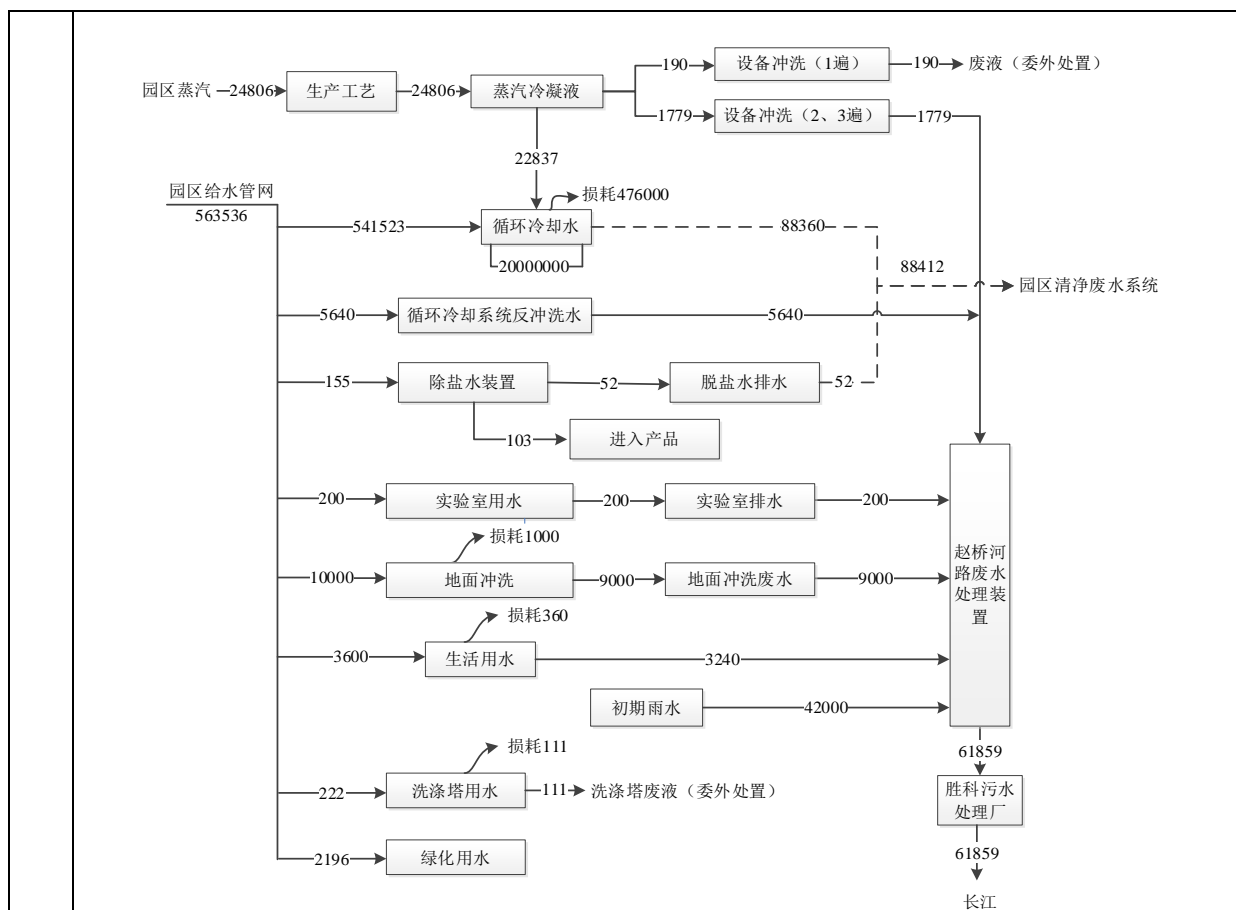
图 2-4 现有项目水平衡图
