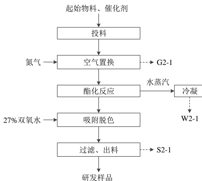
图 2-2 研发实验流程及产污环节图
